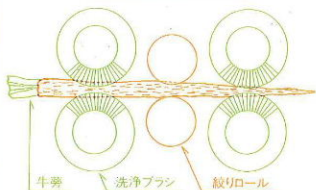
洗浄構造図
