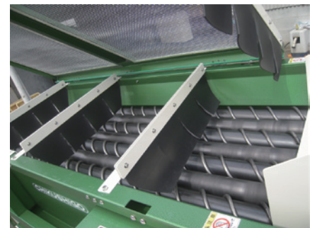
調整機 OTM50-1500
